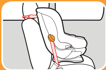
Ceinture sous-abdominale du véhicule avec sangle d'attache supérieure
