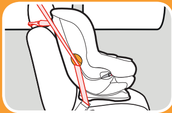
Ceinture sous-abdominale/ diagonale du véhicule avec sangle d'attache supérieure
